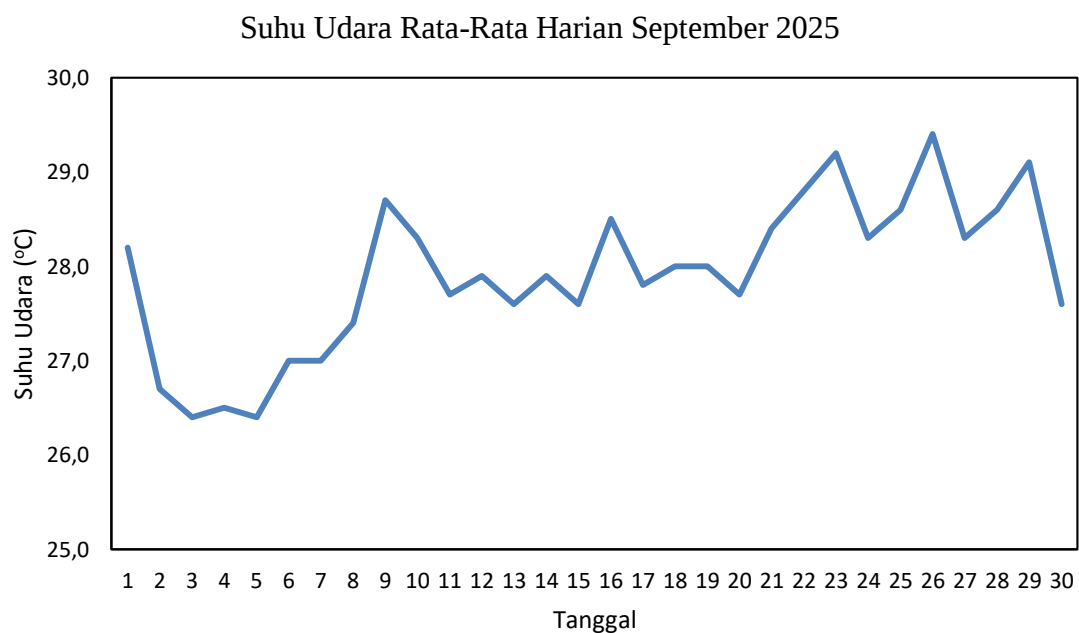
Gambar 2.1 Grafik Suhu Udara Rata-rata Harian Bulan September 2025 di Stasiun Meteorologi Mali - Alor
