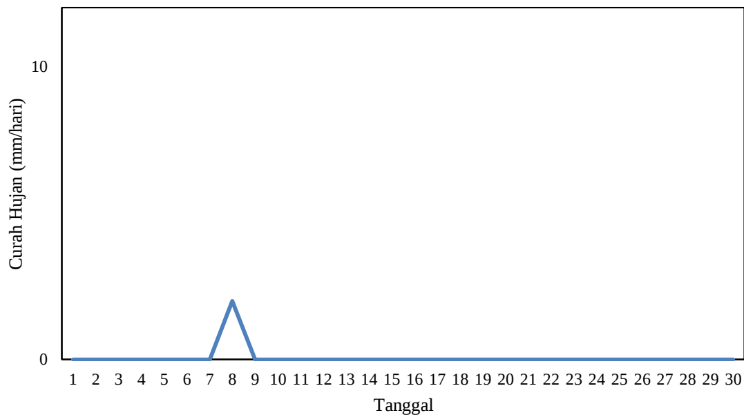
Gambar 2.4 Grafik Curah Hujan Harian September 2025 di Stasiun Meteorologi Mali - Alor
