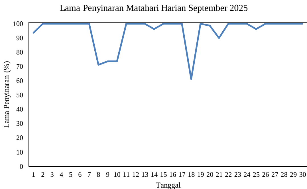
Gambar 2.7 Grafik Lama Penyinaran Matahari Harian bulan September 2025 di Stasiun Meteorologi Mali - Alor
