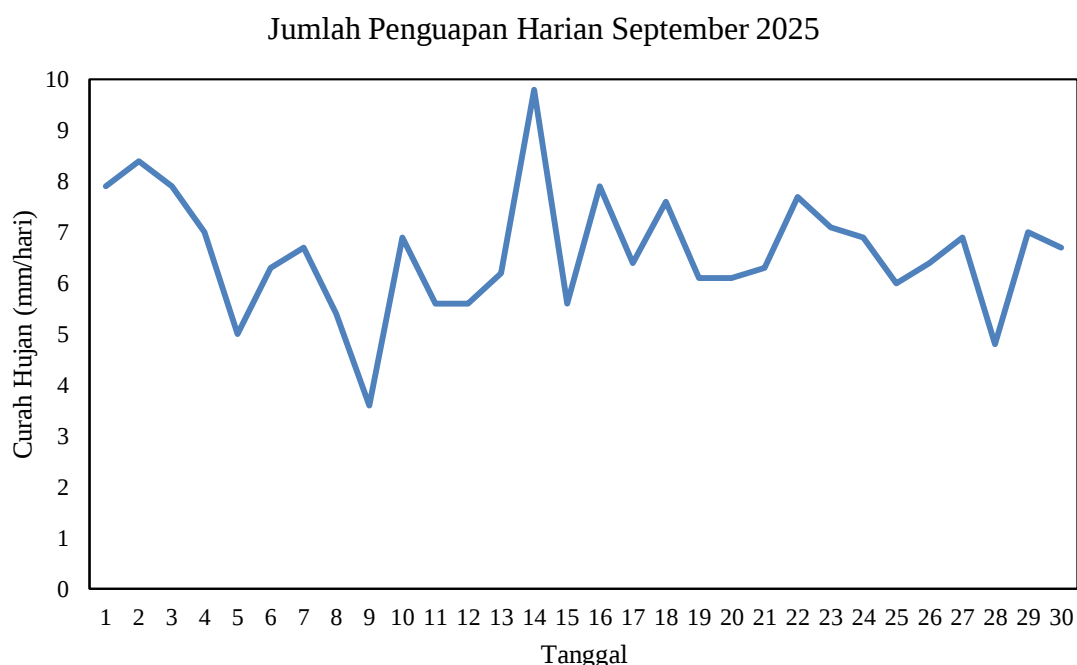
Gambar 2.8 Grafik Jumlah Penguapan Harian bulan September 2025 di Stasiun Meteorologi Mali - Alor
