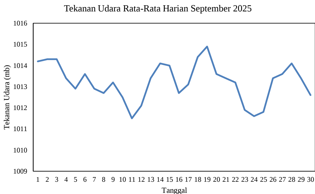
Gambar 2.6 Grafik Tekanan Udara Rata-rata Harian bulan September 2025 di Stasiun Meteorologi Mali - Alor
