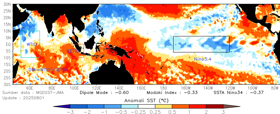
Gambar 3.2 Anomali Suhu Muka Laut di sekitar wilayah Indonesia pada Dasarian V bulan September 2025
