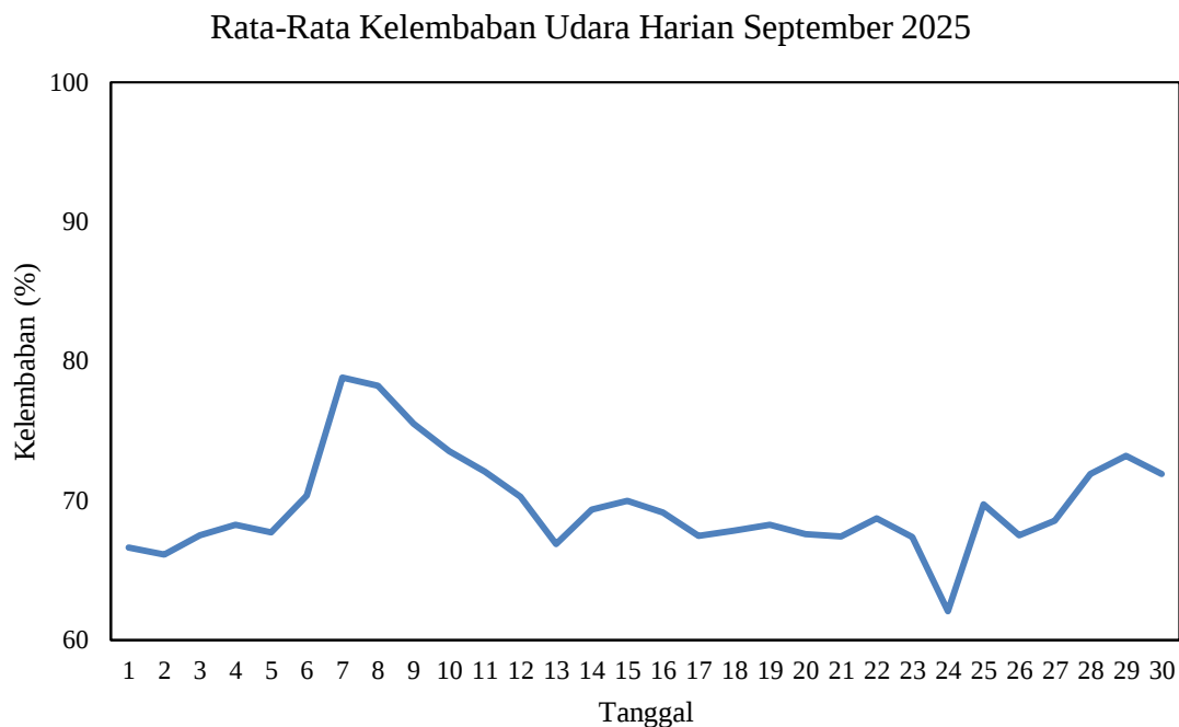
Gambar 2.5 Grafik Rata-rata Kelembaban Udara Harian September 2025 di Stasiun Meteorologi Mali - Alor
