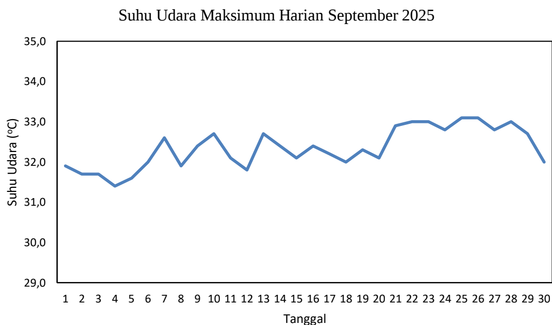
Gambar 2.2 Grafik Suhu Udara Maksimum September 2025 di Stasiun Meteorologi Mali - Alor
