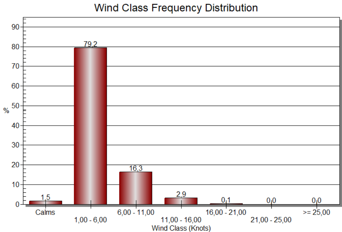
Gambar 2.10 Distribusi Frekuensi Angin Permukaan Bulan September 2025 di Stasiun Meteorologi Mali - Alor
