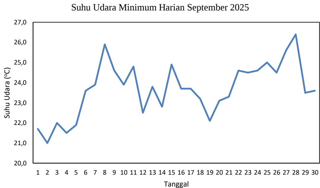
Gambar 2.3 Grafik Suhu Udara Minimum September 2025 di Stasiun Meteorologi Mali - Alor
