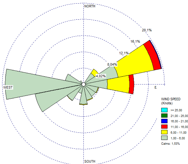
Gambar 2.9 Wind Rose Angin Permukaan Bulan September 2025 di Stasiun Meteorologi Mali - Alor
